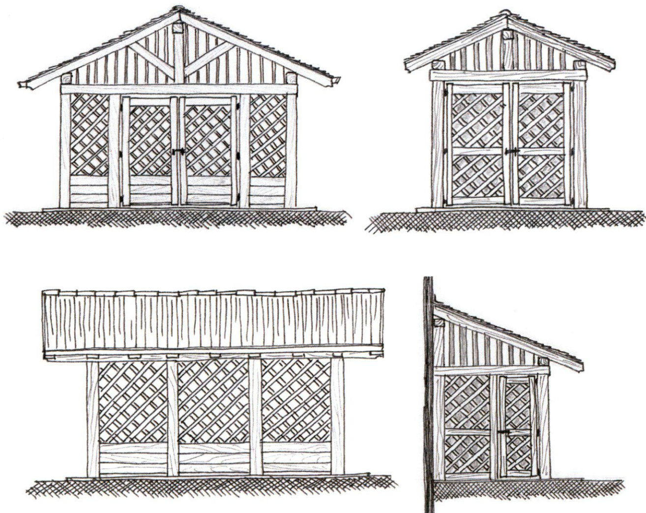
Schema legnaia da preferire nelle zone residenziali
